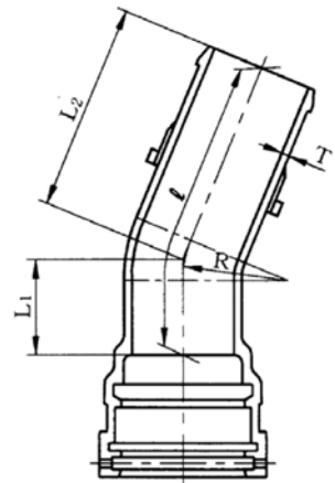
呼び径 75~250
